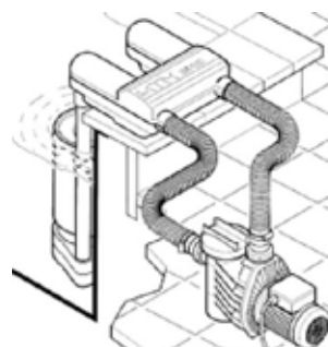
Schwimmskimmer-Set mit Filterinnenteil
