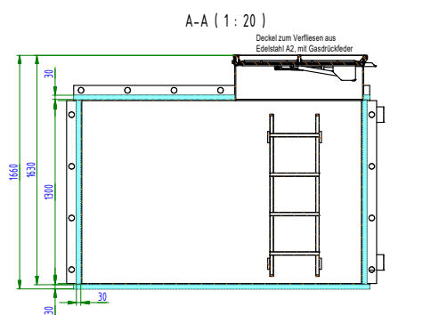
Technikschacht Standard mit Gasdruckfederdeckel 2,0 x 1,5 x 1,3 m
