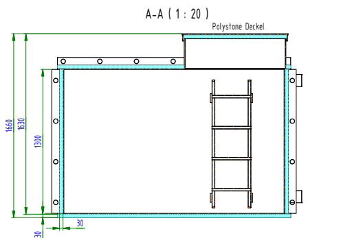
Technikschacht Standard mit Kunststoffdeckel 2,0 x 1,5 x 1,3 m
